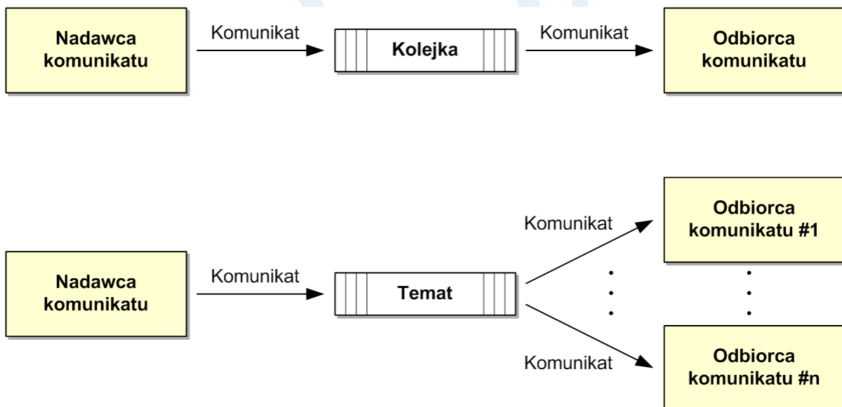
Rys 1. Sposoby asynchronicznego komunikowania się aplikacji z wykorzystaniem systemów kolejkowania
