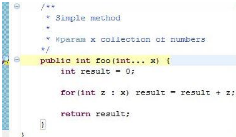
Rysunek 1. Brak taga @return w dokumentacji – informacja wyświetlane przez Eclipse-CS
