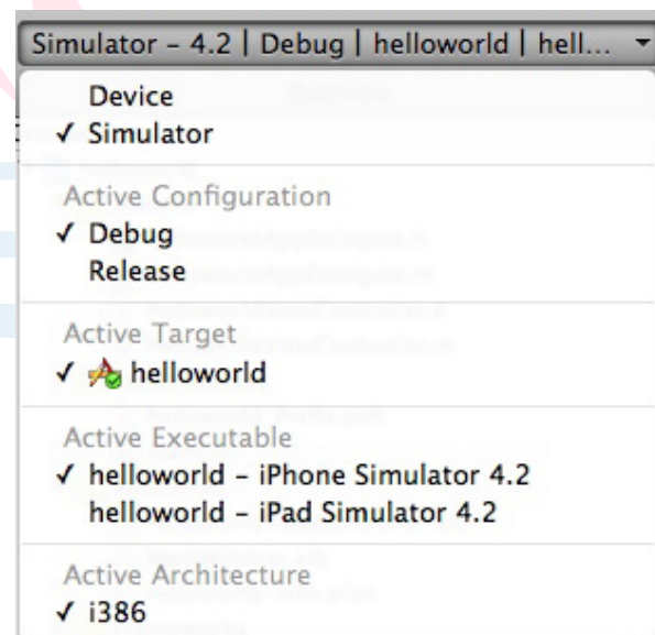
Rys 3. Menu uruchomieniowe
